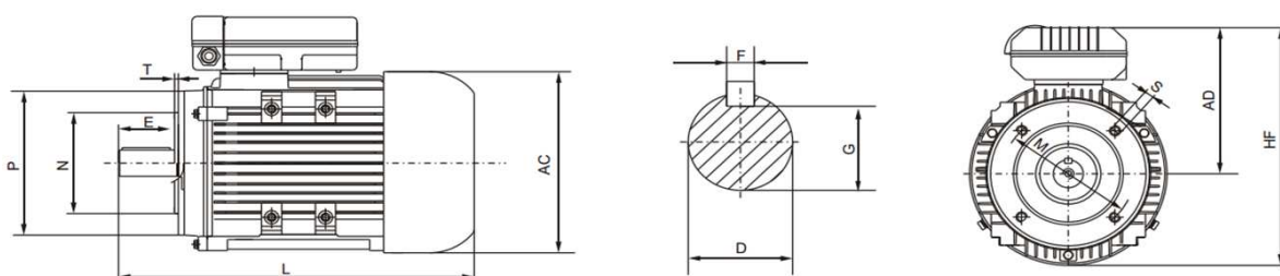
Wymiary silników jednofazowych serii GMY, GMYL oraz GMYC, kołnierowych B14
